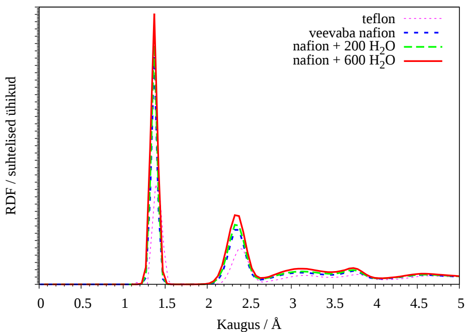
Joonis 5: C8-F8 radiaaljaotusfunktsioonid eri süsteemides
