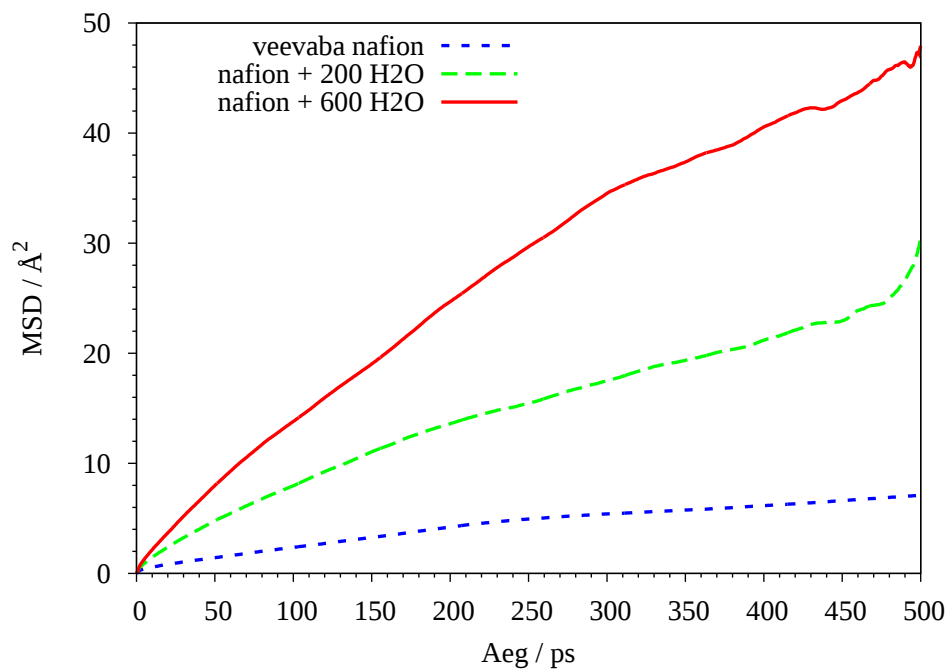
Joonis 18: C5 aatomi MSD eri süsteemides
