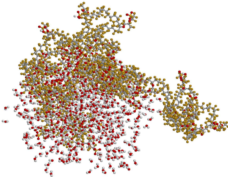
Joonis 6: Neljast Nafioni ja 600 veemolekulist koosnev süsteem pakkimata kujul enne simulatsiooni.
