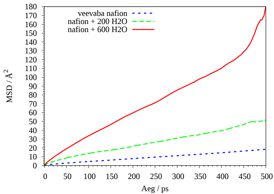
Joonis 22: H1 aatomi MSD eri süsteemides
