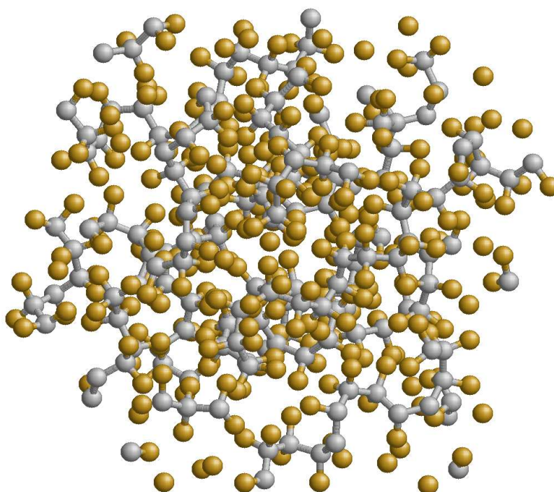
Joonis 2: Tefloni molekul simulatsioonirakku pakituna pärast simulatsiooni.
