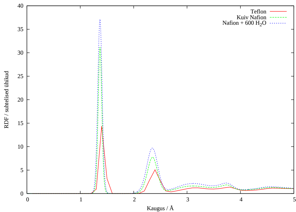
Joonis 10: C8-F8 radiaaljaotusfunktsioonid eri süsteemides
