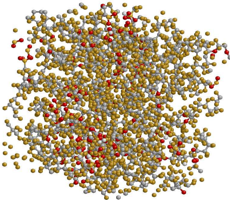
Joonis 5: Simulatsioonirakk veevaba Nafioniga pärast simulatsiooni.
