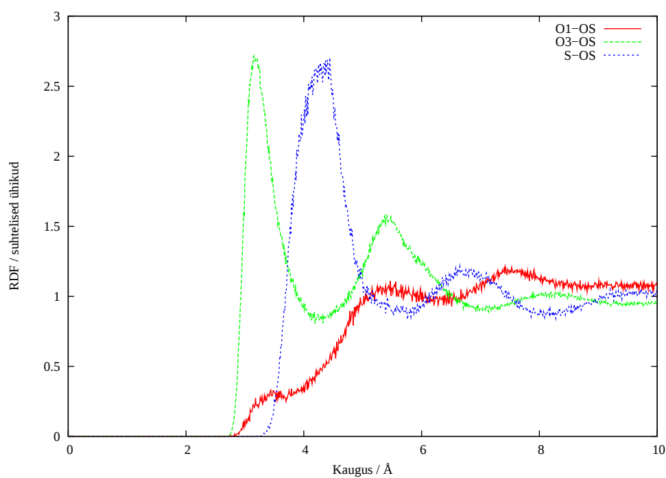
Joonis 11: Nafion + 600 H 2 O radiaaljaotusfunktsioonid
