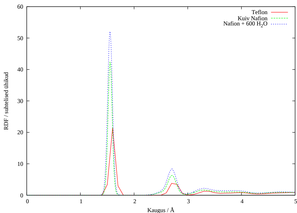
Joonis 9: C8-C8 radiaaljaotusfunktsioonid eri süsteemides
