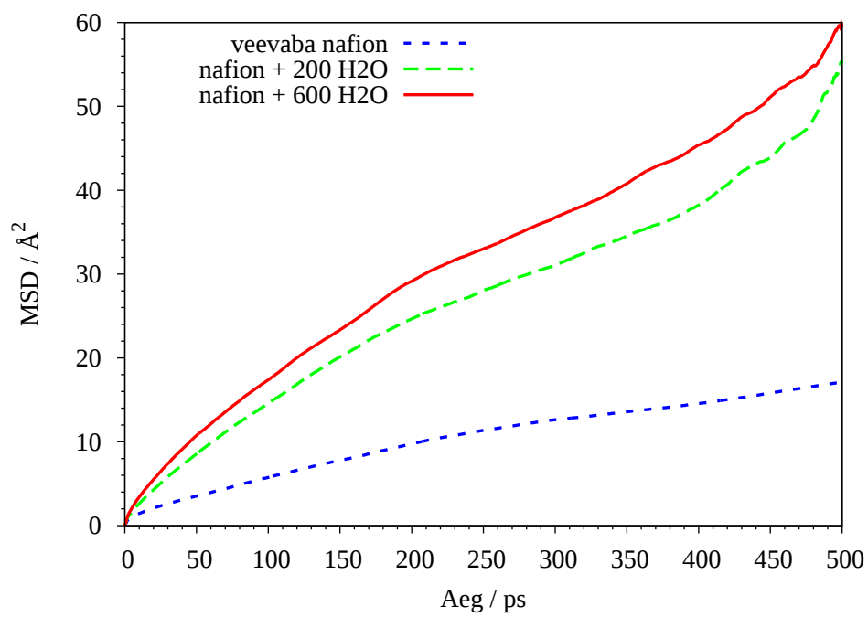
Joonis 15: F3 aatomi MSD eri süsteemides
