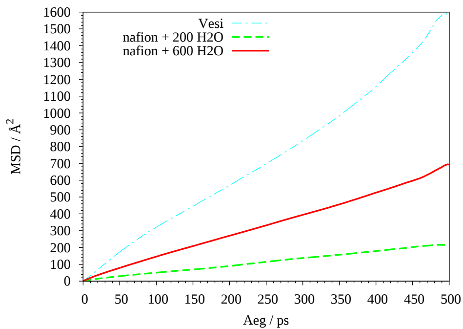
Joonis 23: OS aatomi MSD eri süsteemides
