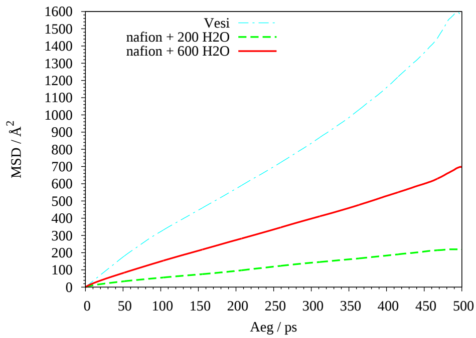
Joonis 24: HW aatomi MSD eri süsteemides
