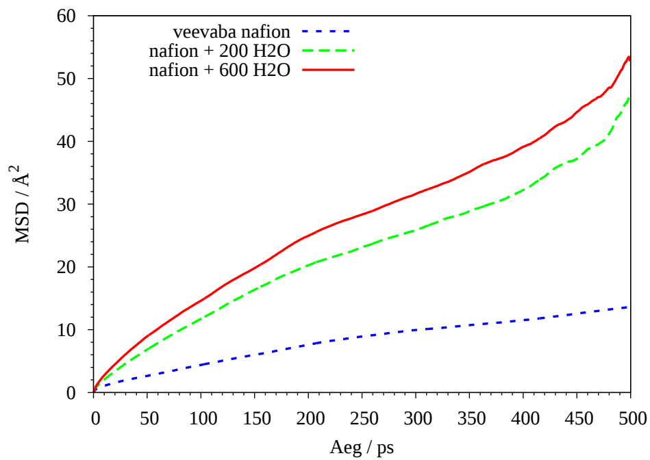
Joonis 14: C3 aatomi MSD eri süsteemides
