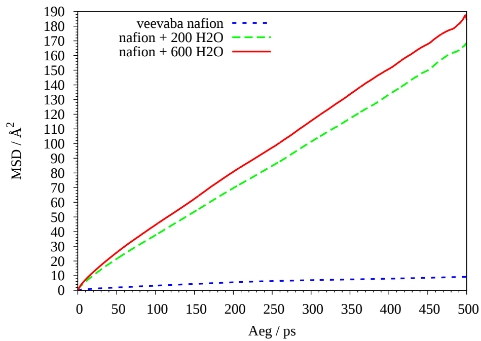
Joonis 21: O3 aatomi MSD eri süsteemides
