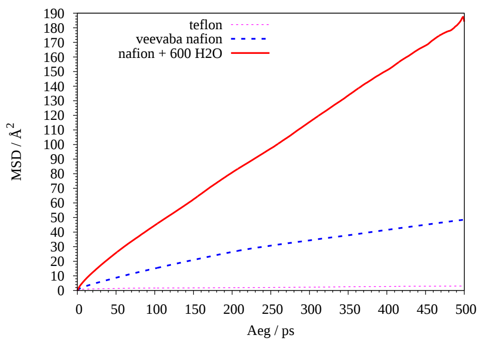
Joonis 13: F8 aatomi MSD eri süsteemides
