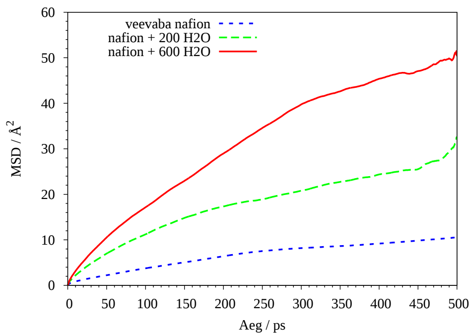
Joonis 19: F5 aatomi MSD eri süsteemides
