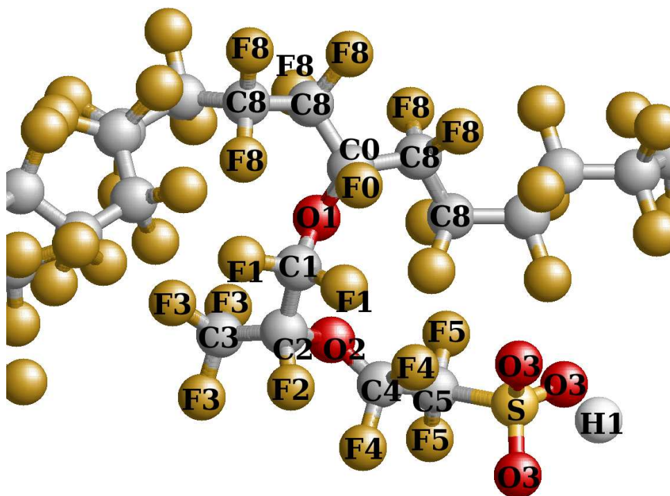
Joonis 3: Lõik nafioni® ahelast. Aatomid C8 ja F8 kuuluvad peaahelasse, ülejäänud kõrvalahelasse.
