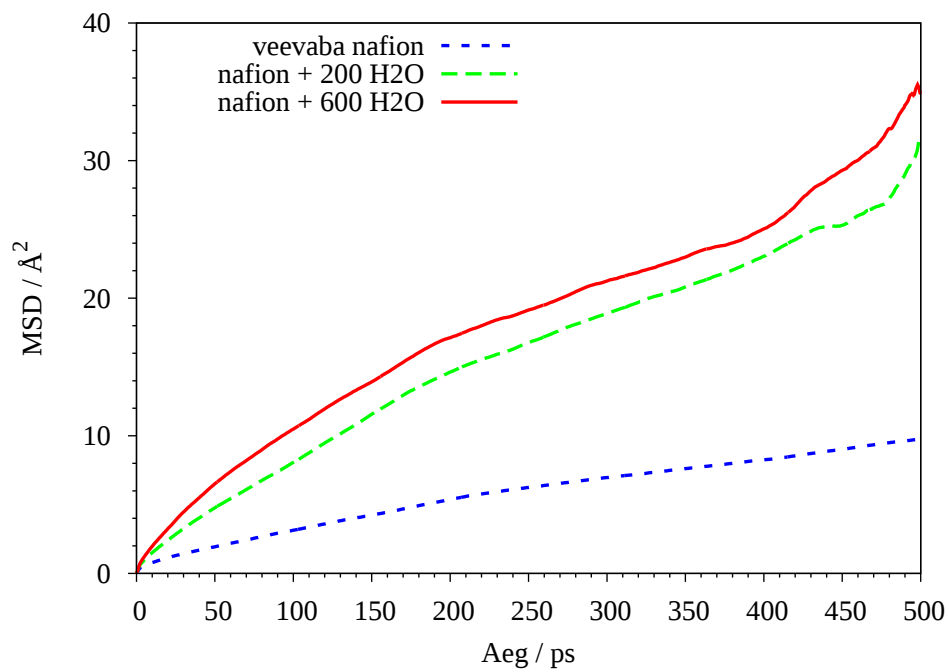
Joonis 16: C1 aatomi MSD eri süsteemides
