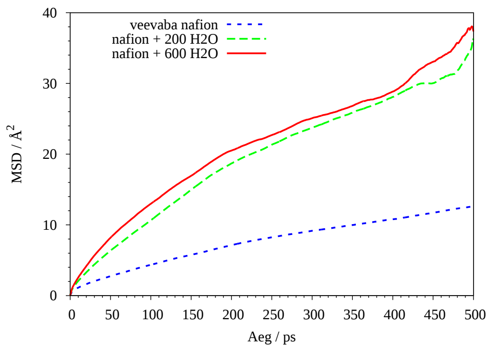
Joonis 17: F1 aatomi MSD eri süsteemides
