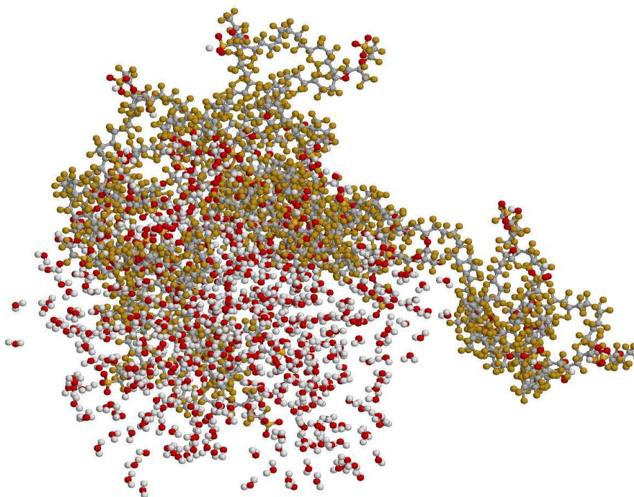
Joonis 5: Neljast Nafioni ja 600 veemolekulist koosnev süsteem pakkimata kujul enne simulatsiooni.
