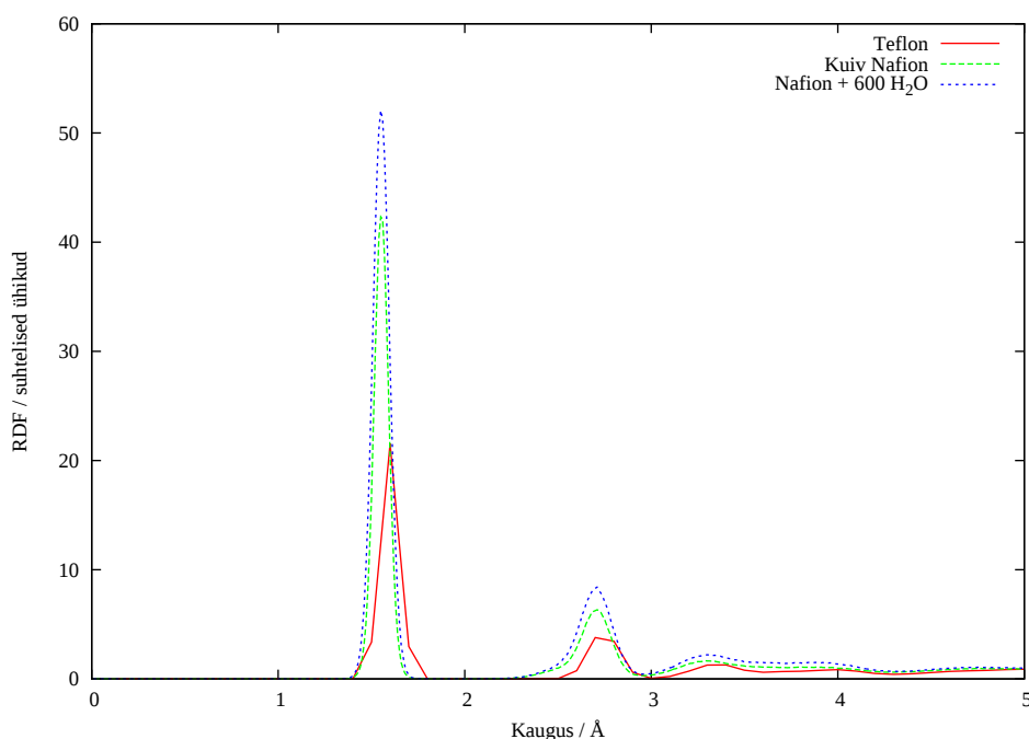
Joonis 8: C8-C8 radiaaljaotusfunktsioonid eri süsteemides
