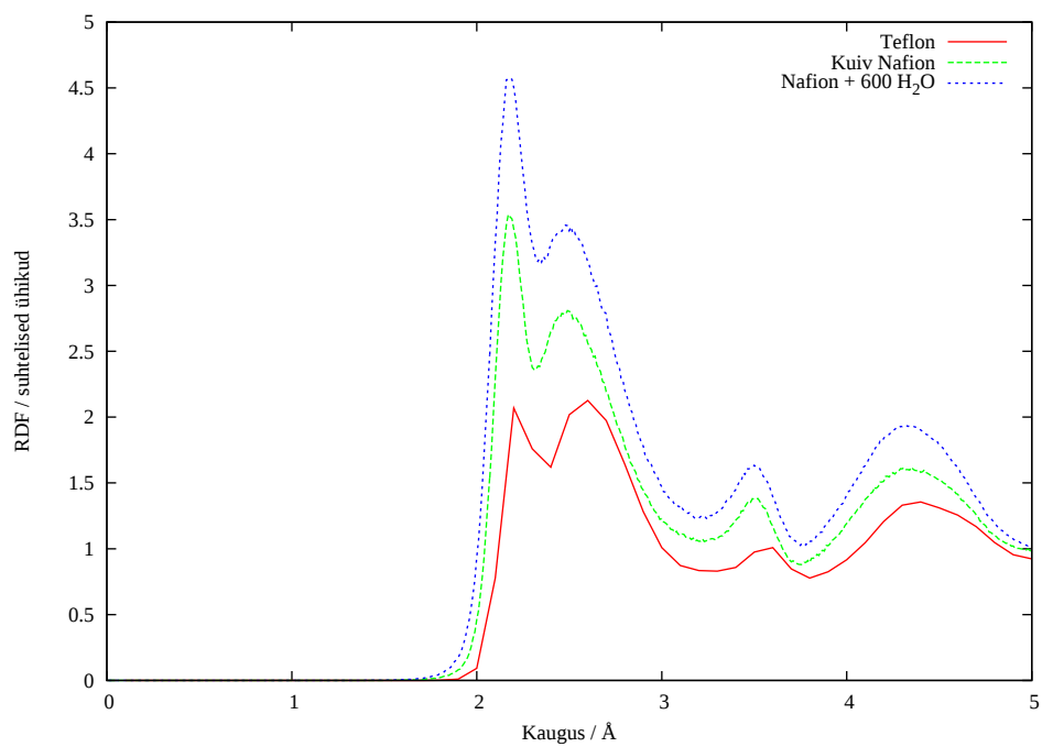
Joonis 10: F8-F8 radiaaljaotusfunktsioonid eri süsteemides
