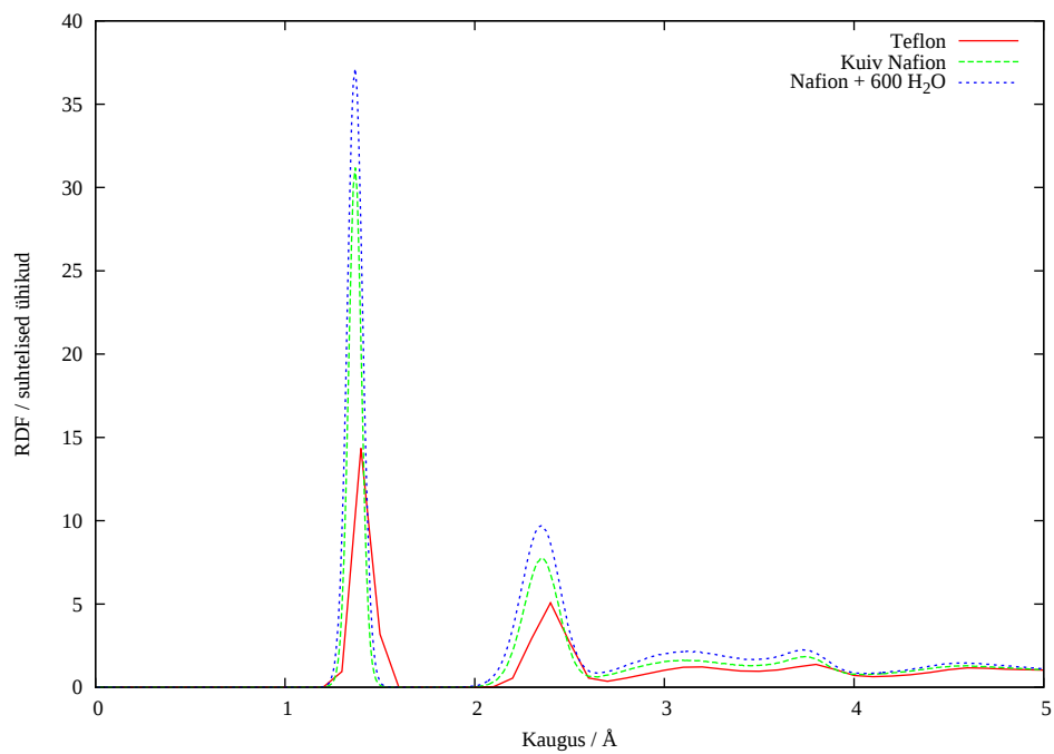
Joonis 9: C8-F8 radiaaljaotusfunktsioonid eri süsteemides
