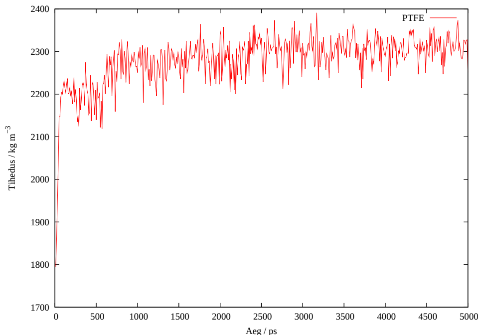
Joonis 7: Modelleeritud Tefloni tiheduse ajaline käik
