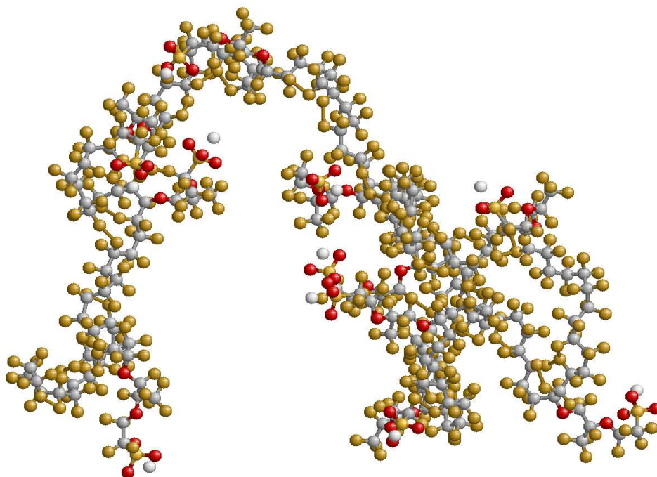
Joonis 3: Üks Nafioni ahel pakkimata kujul enne simulatsiooni.
