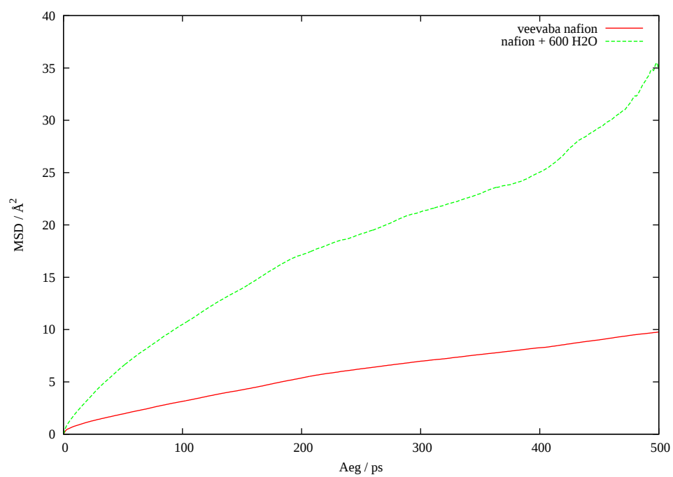
Joonis 12: C1 aatomi MSD eri süsteemides
