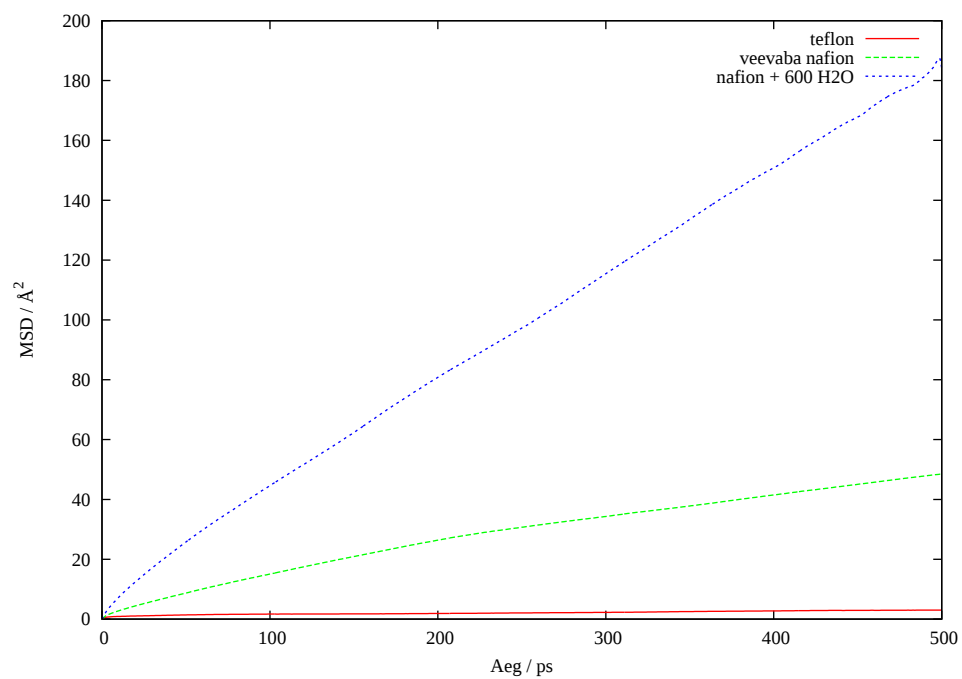
Joonis 9: F8 aatomi MSD eri süsteemides
