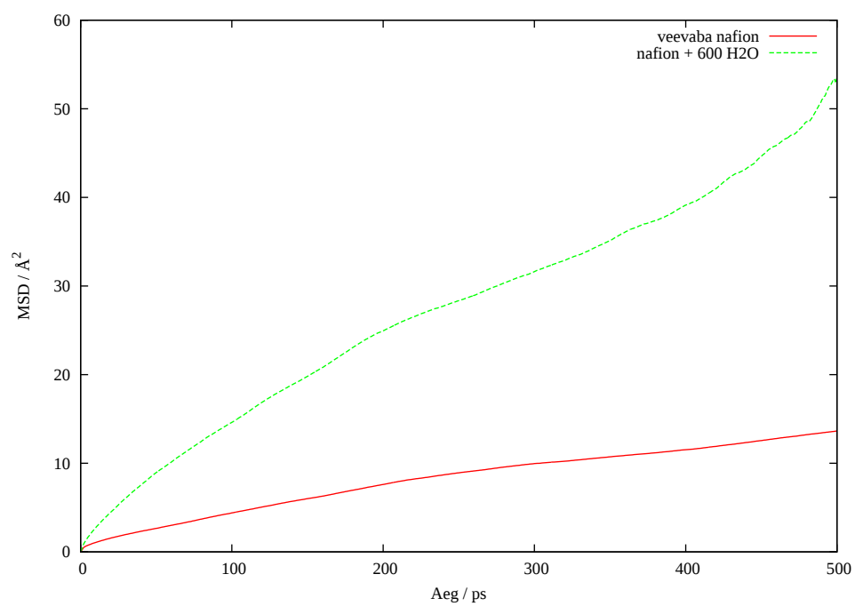
Joonis 10: C3 aatomi MSD eri süsteemides
