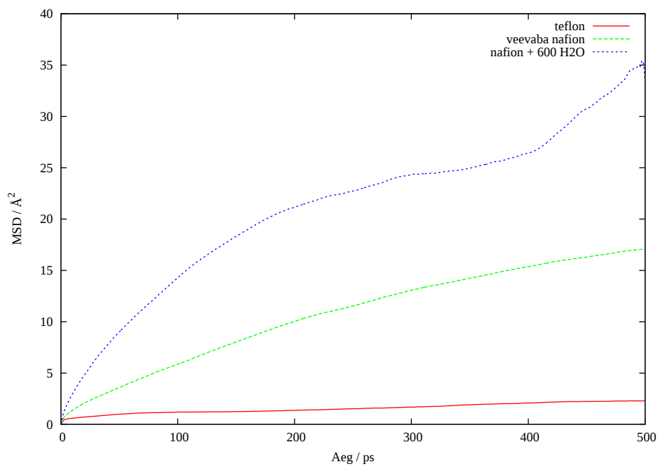
Joonis 8: C8 aatomi MSD eri süsteemides
