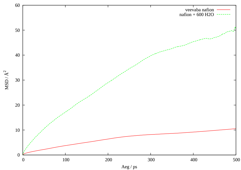
Joonis 15: F5 aatomi MSD eri süsteemides
