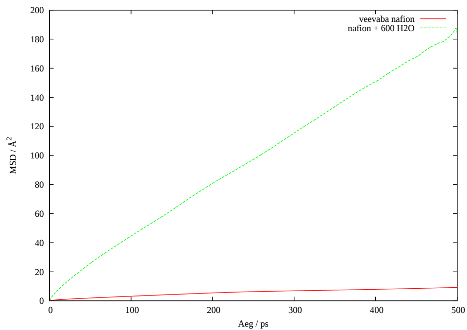
Joonis 17: O3 aatomi MSD eri süsteemides
