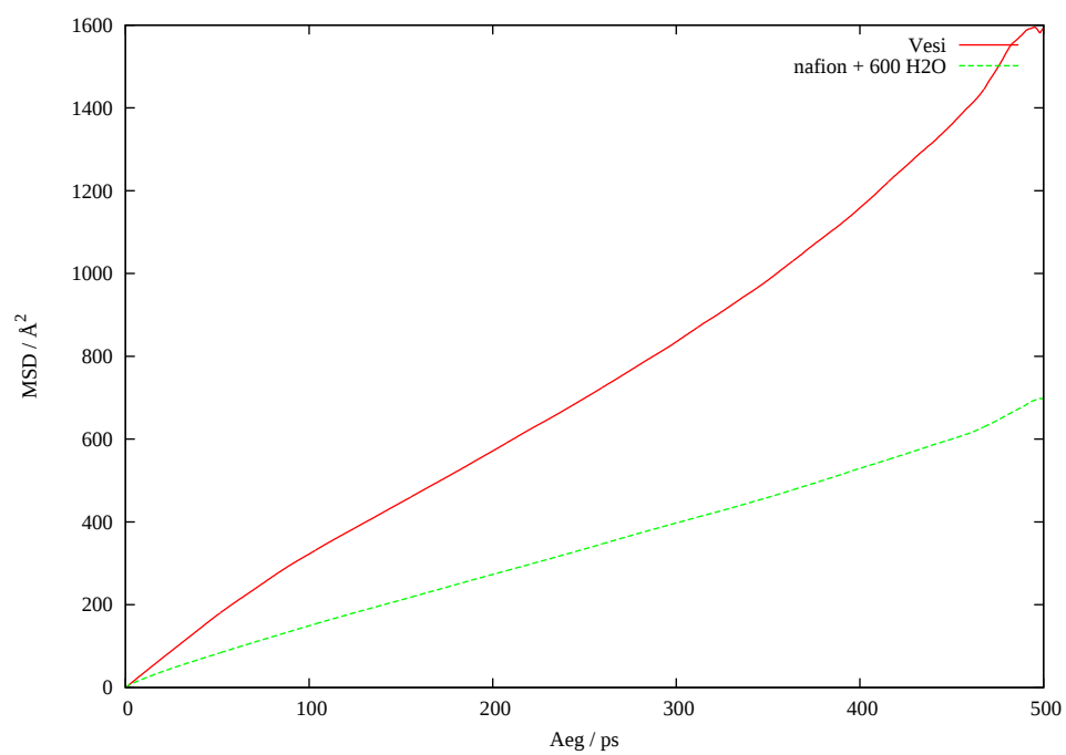
Joonis 20: HW aatomi MSD eri süsteemides
