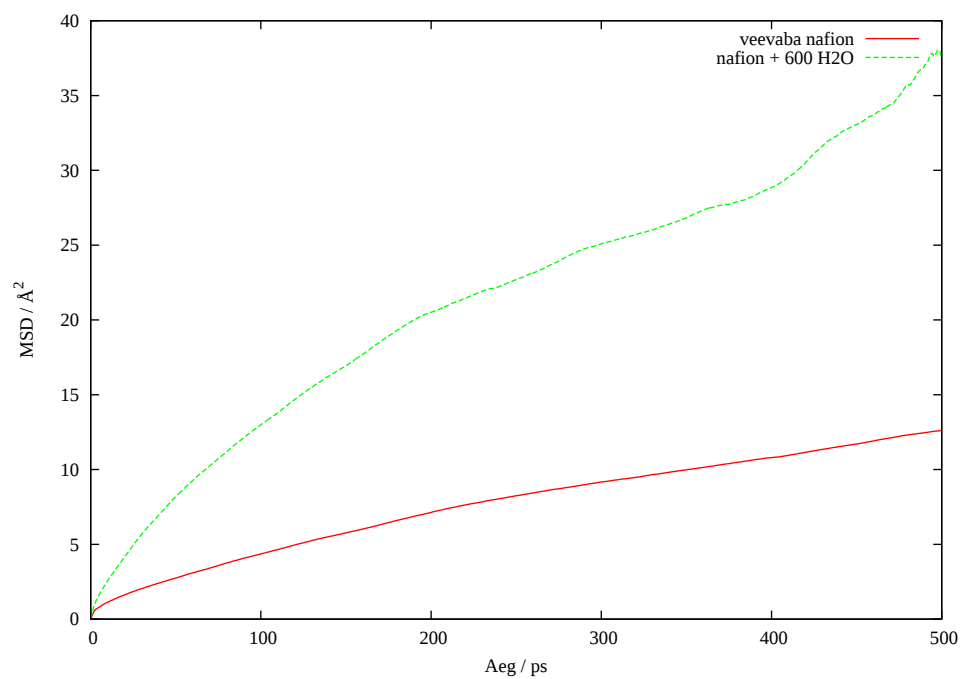
Joonis 13: F1 aatomi MSD eri süsteemides
