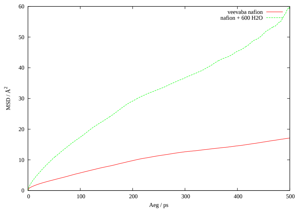
Joonis 11: F3 aatomi MSD eri süsteemides
