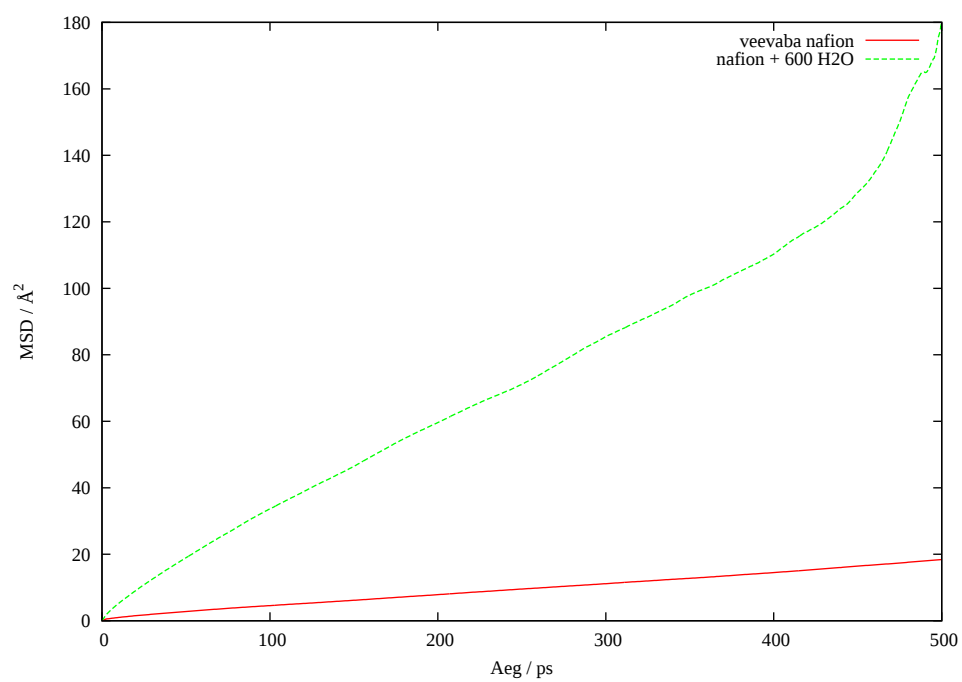
Joonis 18: H1 aatomi MSD eri süsteemides
