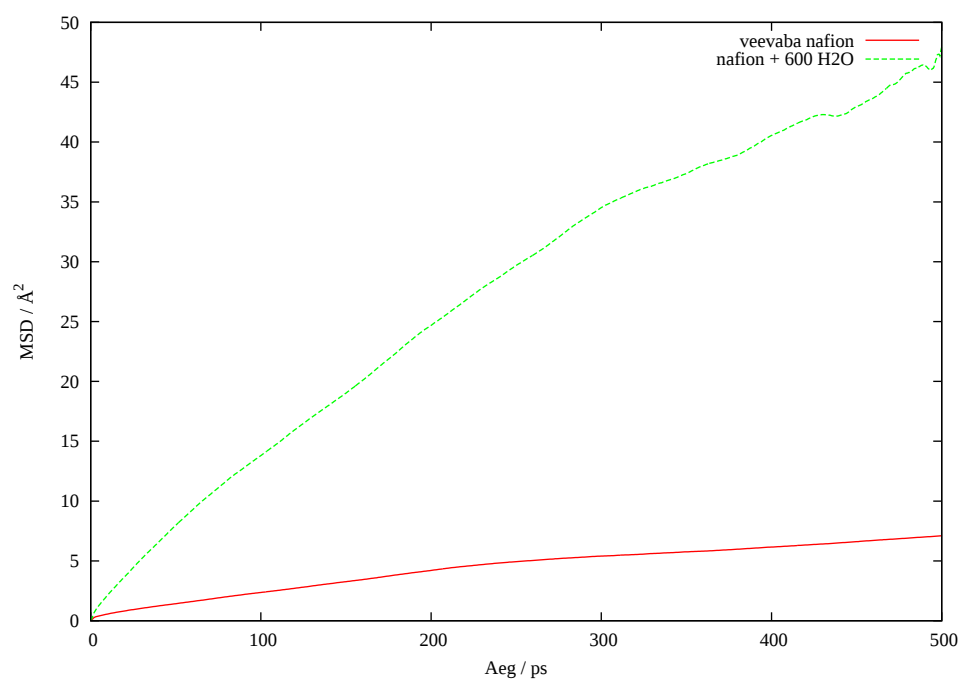
Joonis 14: C5 aatomi MSD eri süsteemides
