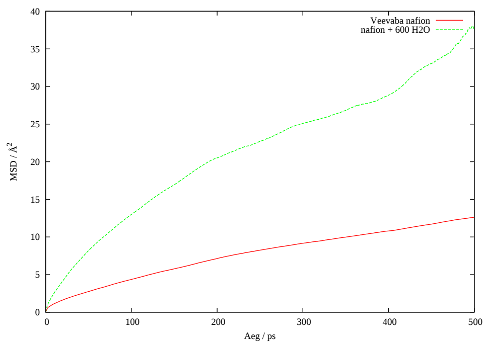
Joonis 12: F1 aatomi MSD eri süsteemides
