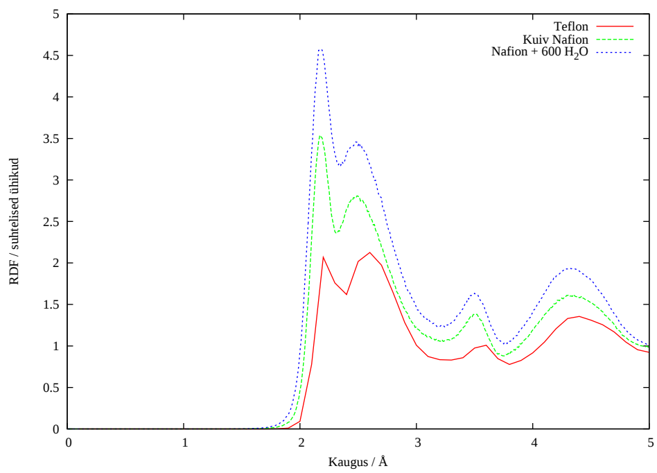
Joonis 6: F8-F8 radiaaljaotusfunktsioonid eri süsteemides
