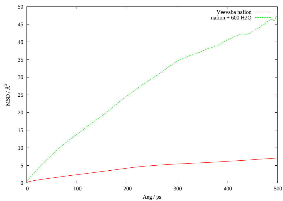
Joonis 10: C5 aatomi MSD eri süsteemides
