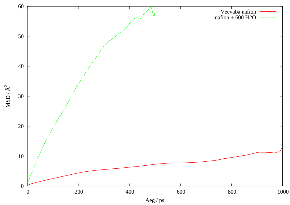
Joonis 20: S aatomi MSD eri süsteemides
