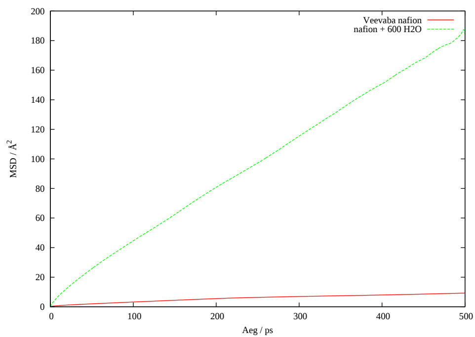
Joonis 18: O3 aatomi MSD eri süsteemides
