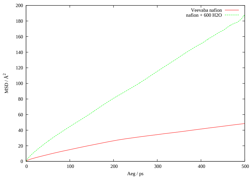
Joonis 15: F8 aatomi MSD eri süsteemides
