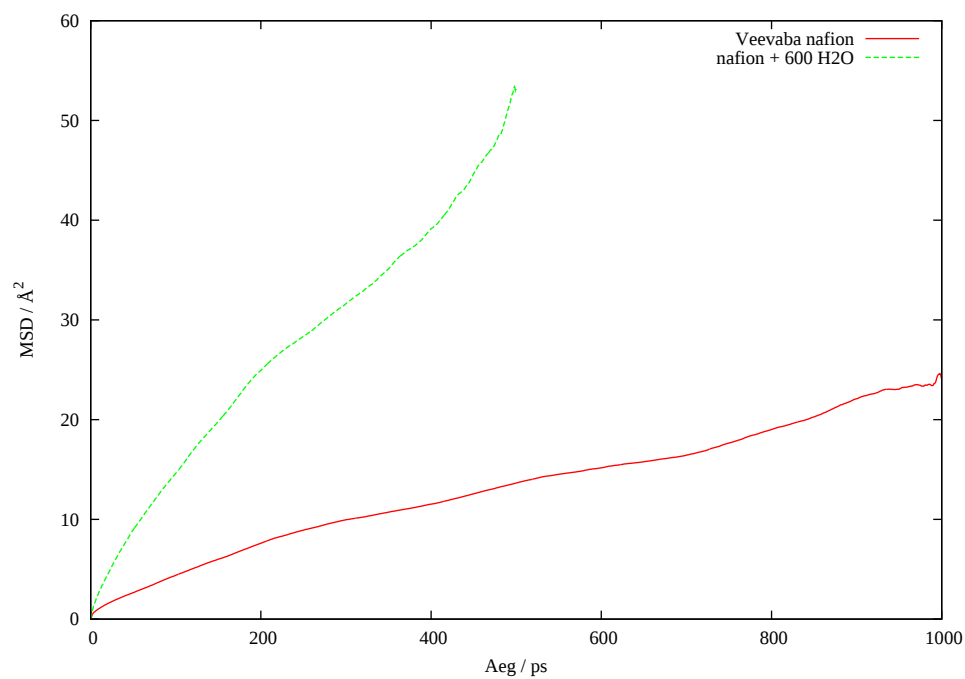
Joonis 9: C3 aatomi MSD eri süsteemides
