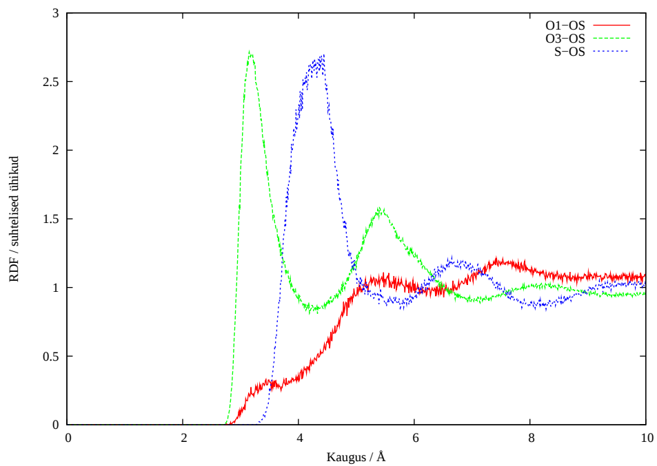
Joonis 7: Nafion + 600 H 2 O radiaaljaotusfunktsioonid
