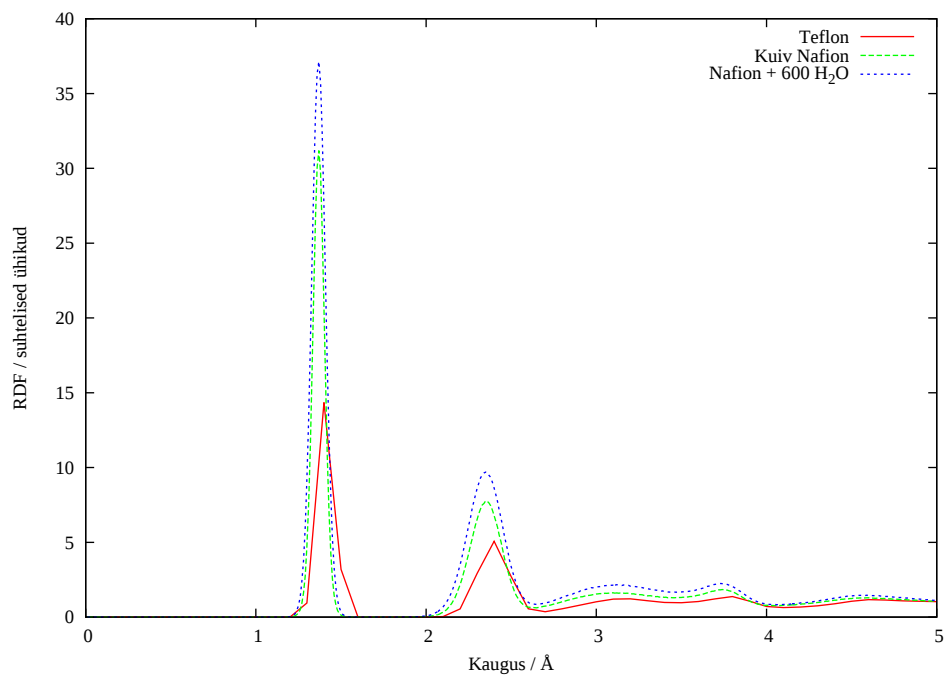
Joonis 5: C8-F8 radiaaljaotusfunktsioonid eri süsteemides
