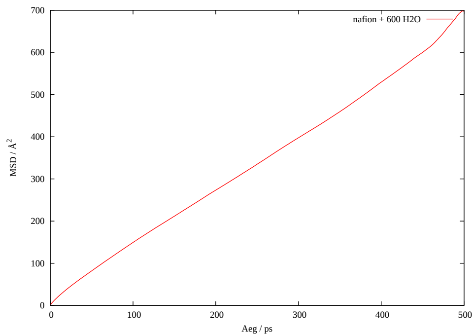
Joonis 17: HW aatomi MSD eri süsteemides
