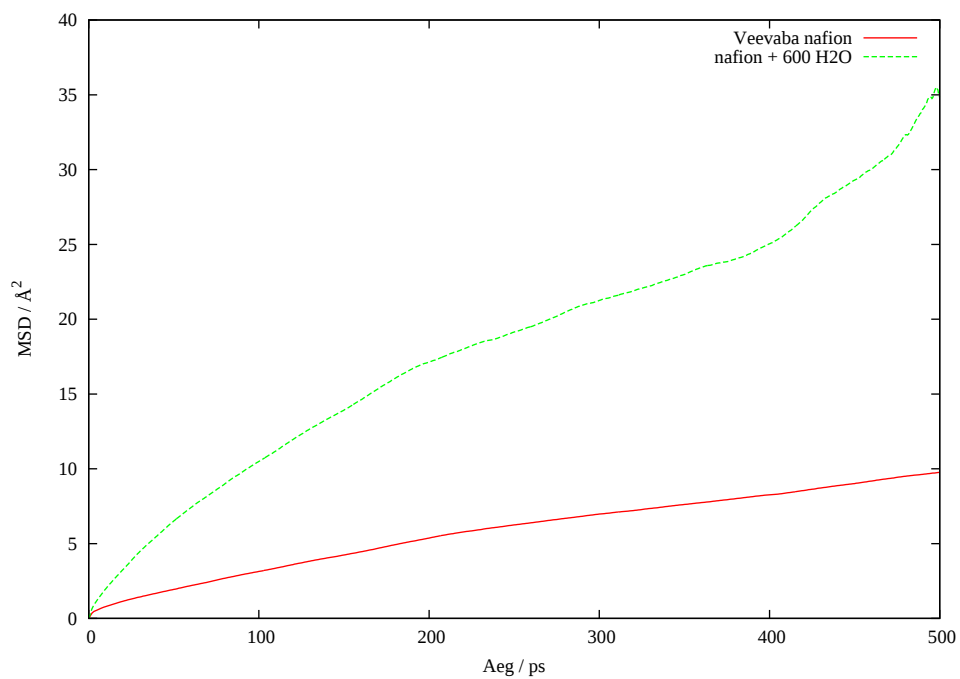
Joonis 8: C1 aatomi MSD eri süsteemides
