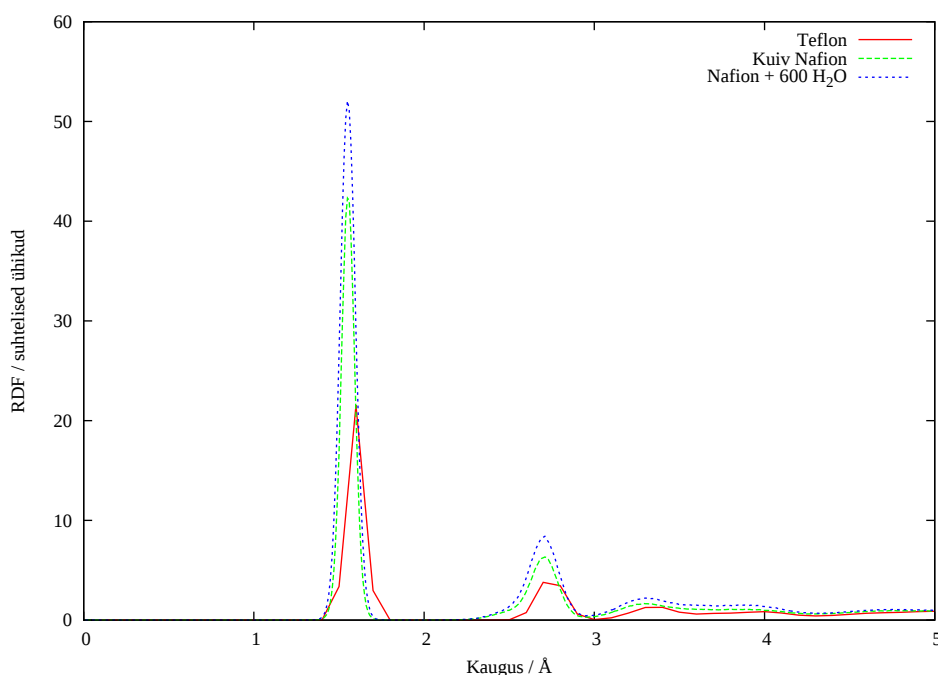
Joonis 4: C8-C8 radiaaljaotusfunktsioonid eri süsteemides
