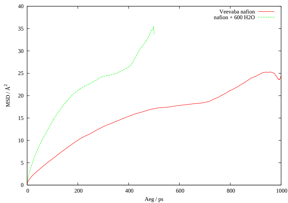
Joonis 11: C8 aatomi MSD eri süsteemides
