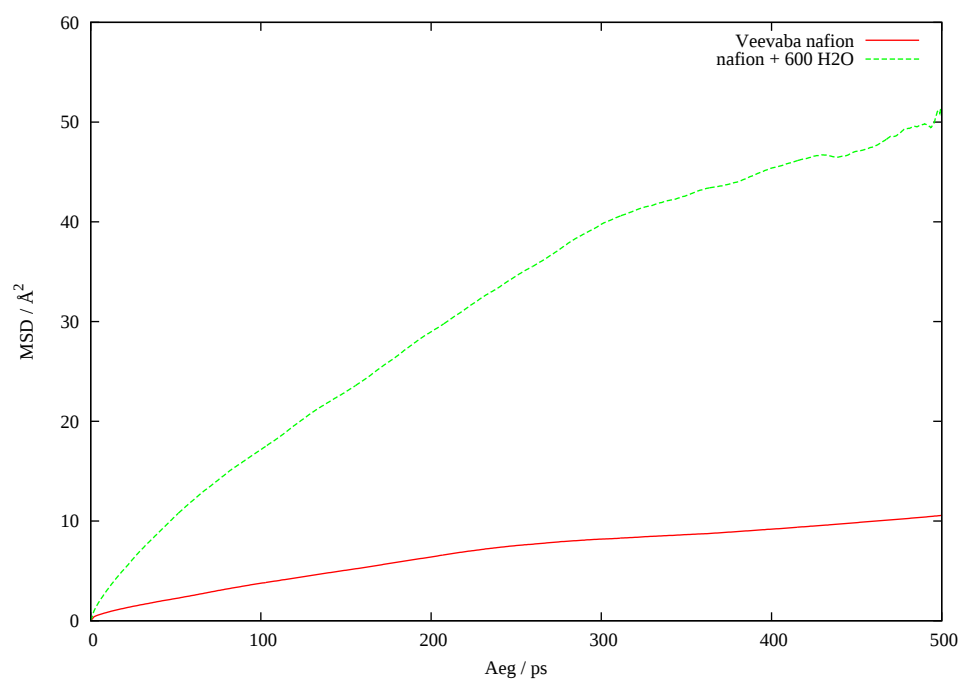
Joonis 14: F5 aatomi MSD eri süsteemides
