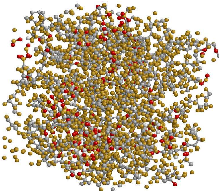
Joonis 2: Simulatsioonirakk veevaba Nafioniga pärast simulatsiooni.
