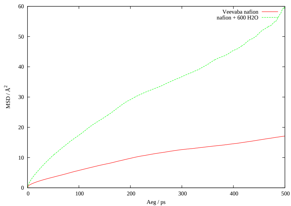
Joonis 13: F3 aatomi MSD eri süsteemides
