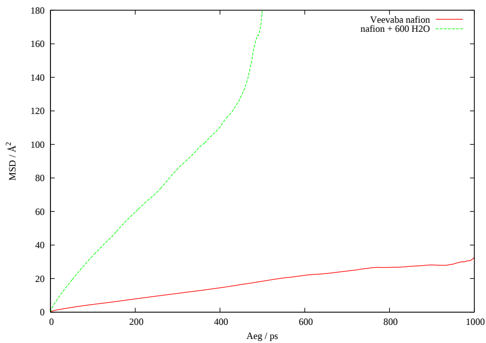
Joonis 16: H1 aatomi MSD eri süsteemides
