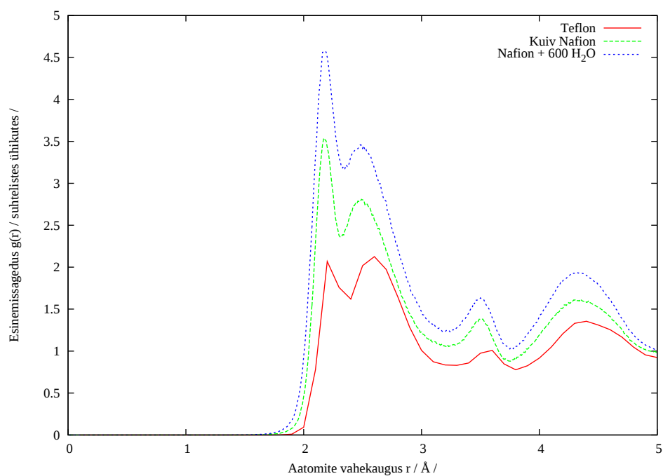
Joonis 7: F8-F8 radiaaljaotusfunktsioonid eri süsteemides
