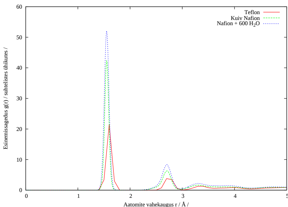
Joonis 5: C8-C8 radiaaljaotusfunktsioonid eri süsteemides
