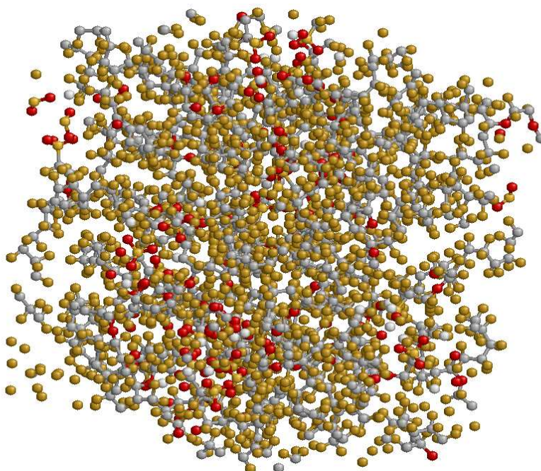
Joonis 3: Simulatsioonirakk veevaba Nafioniga pärast simulatsiooni.
