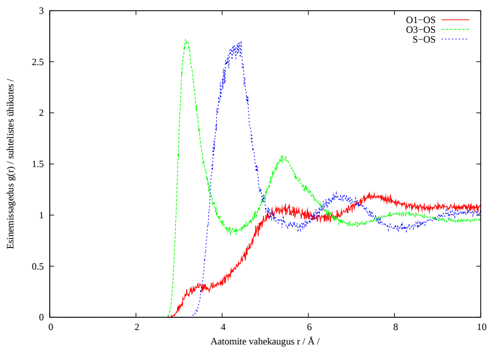
Joonis 8: Nafion + 600 H 2 O radiaaljaotusfunktsioonid
