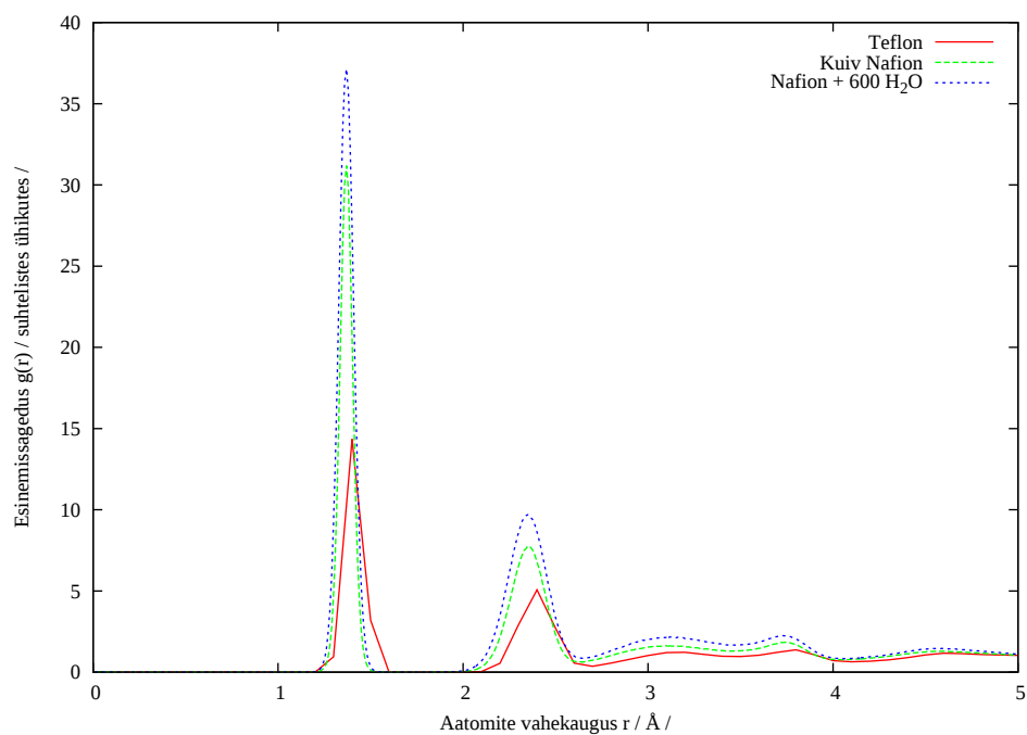
Joonis 6: C8-F8 radiaaljaotusfunktsioonid eri süsteemides
