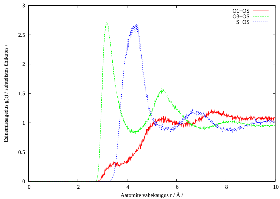
Joonis 9: Nafion + 600 H 2 O radiaaljaotusfunktsioonid
