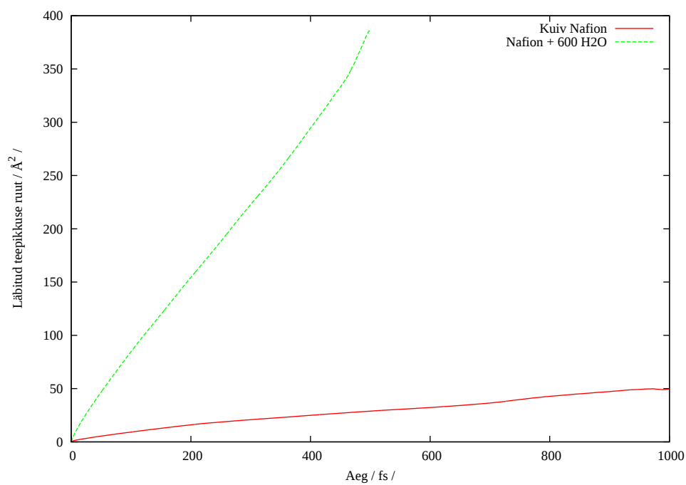
Joonis 10: C3 MSD-funktsioonid eri süsteemides
