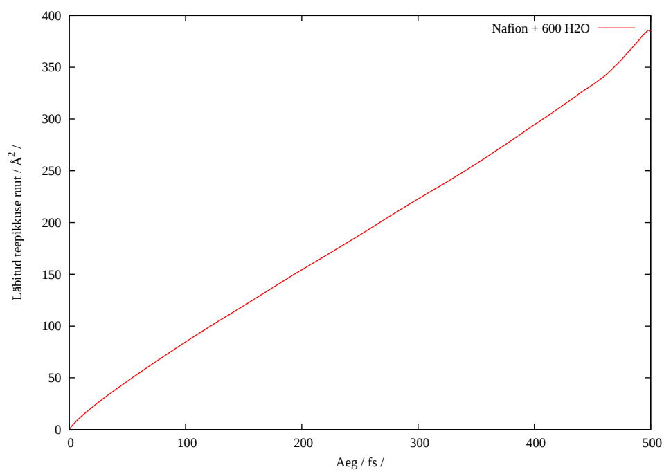
Joonis 14: OS MSD-funktsioon Nafion + 600 H2O süsteemis
