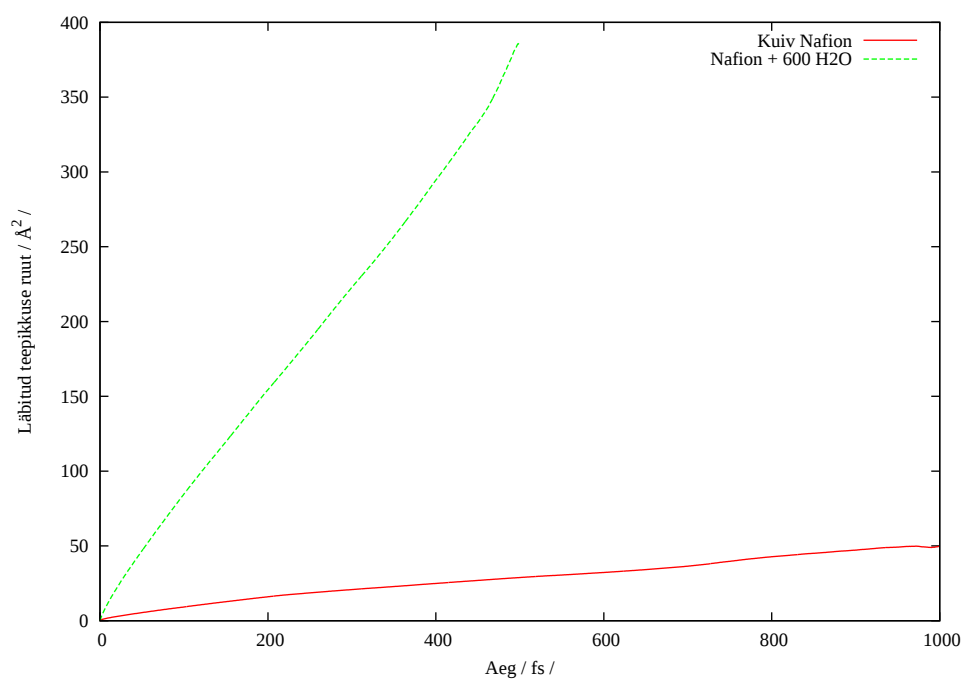
Joonis 12: Vesinikuiooni MSD-funktsioonid eri süsteemides
