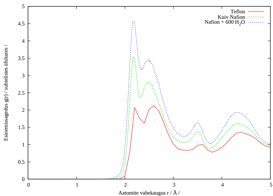
Joonis 8: F8-F8 radiaaljaotusfunktsioonid eri süsteemides
