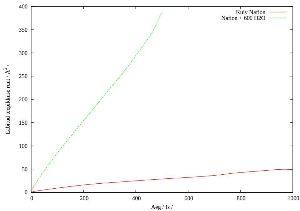
Joonis 11: C8 MSD-funktsioonid eri süsteemides
