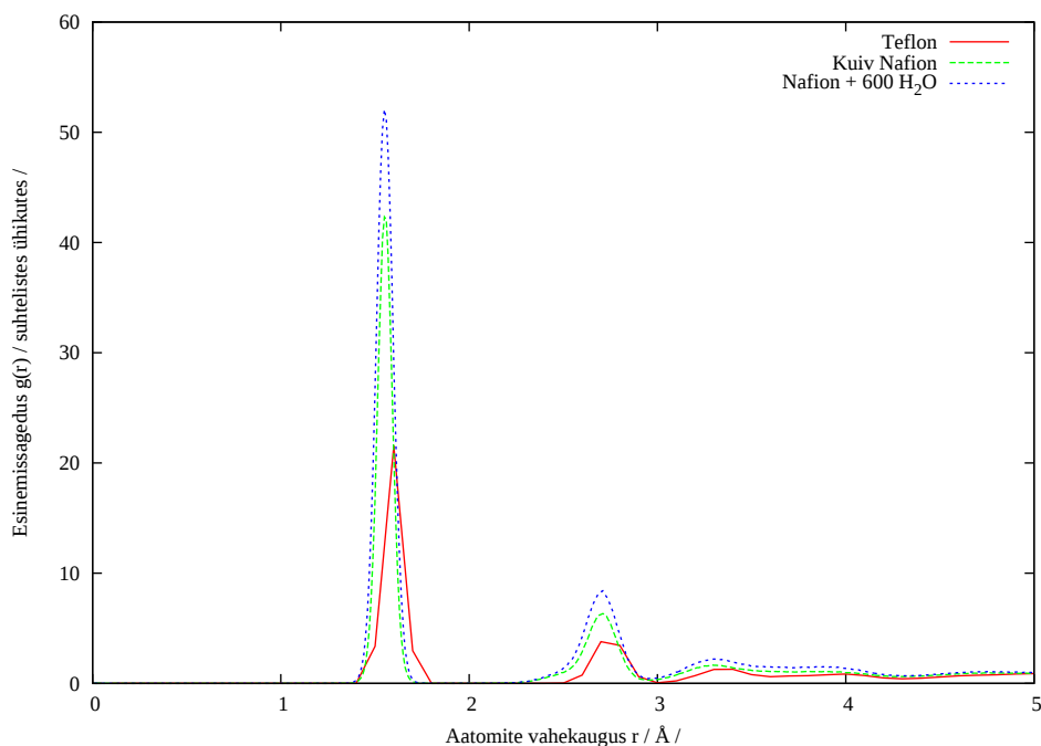
Joonis 6: C8-C8 radiaaljaotusfunktsioonid eri süsteemides
