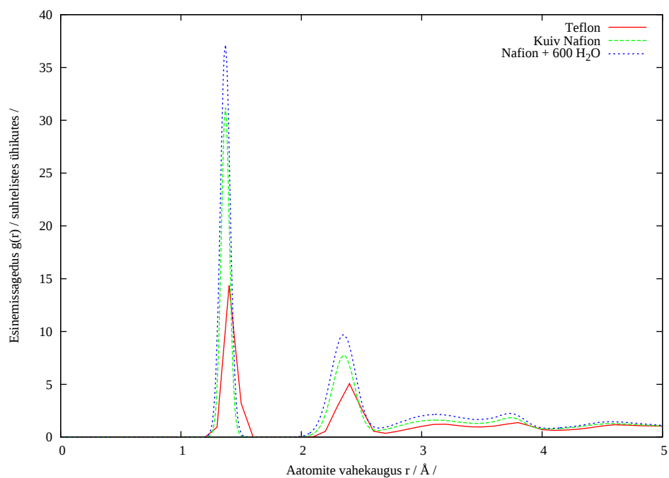
Joonis 7: C8-F8 radiaaljaotusfunktsioonid eri süsteemides
