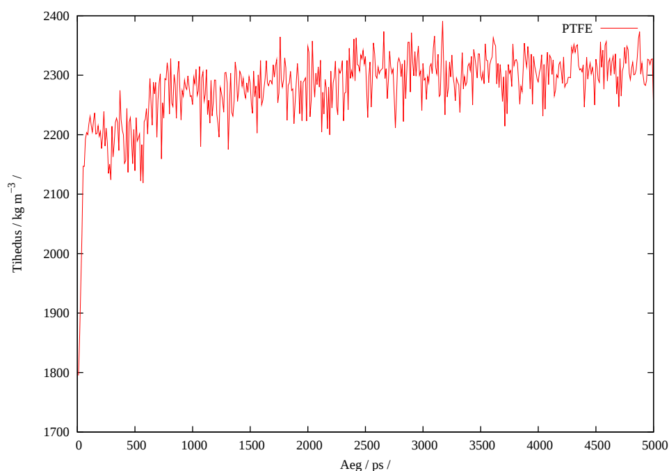
Joonis 5: Modelleeritud Tefloni tiheduse ajaline käik
