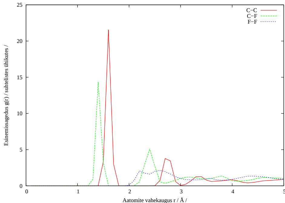
Joonis 4: Modelleeritud Tefloni radiaaljaotusfunktsioon
