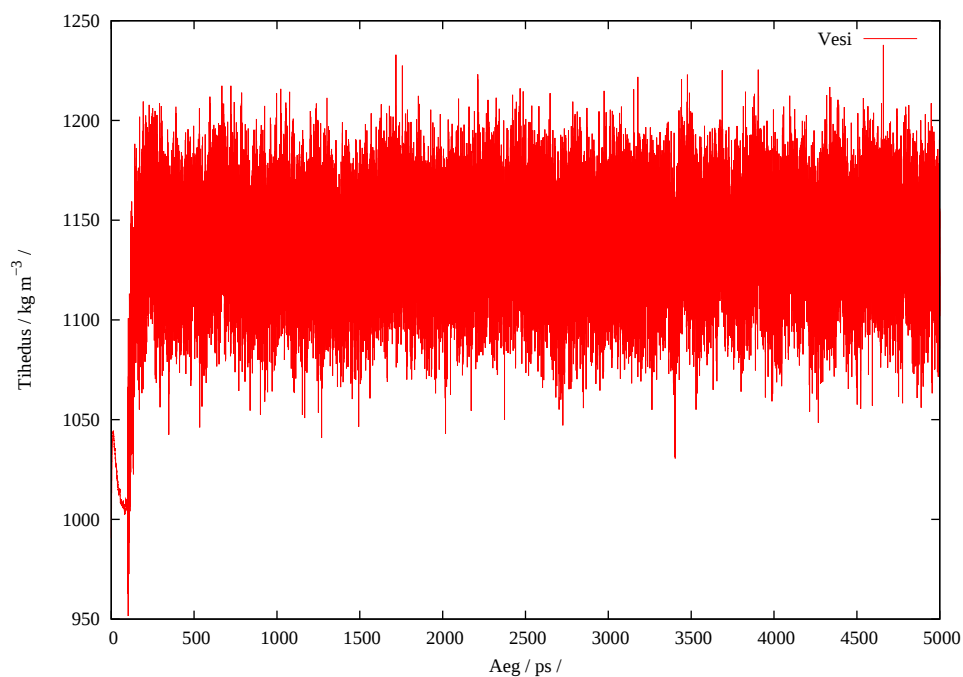
Joonis 8: Modelleeritud vee tiheduse ajaline käik
