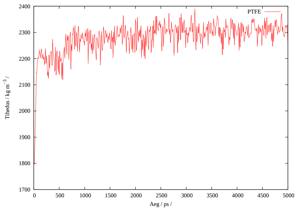
Joonis 6: Modelleeritud Tefloni tiheduse ajaline käik
