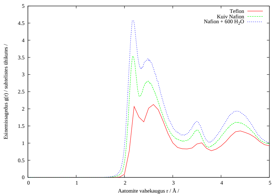
Joonis 11: F8-F8 radiaaljaotusfunktsioonid eri süsteemides
