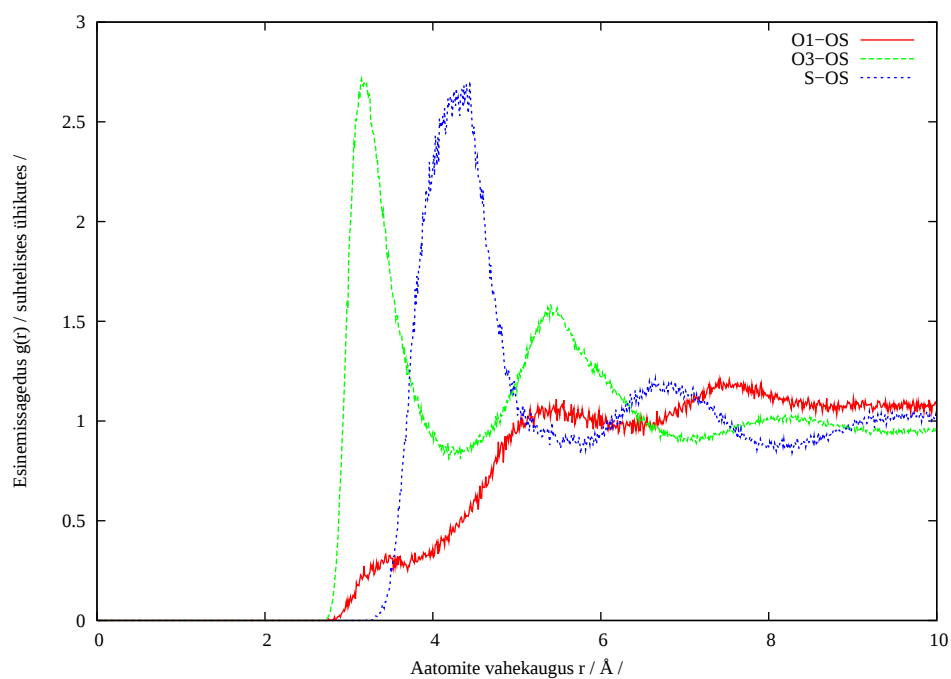
Joonis 12: Nafion + 600 H 2 O radiaaljaotusfunktsioonid
