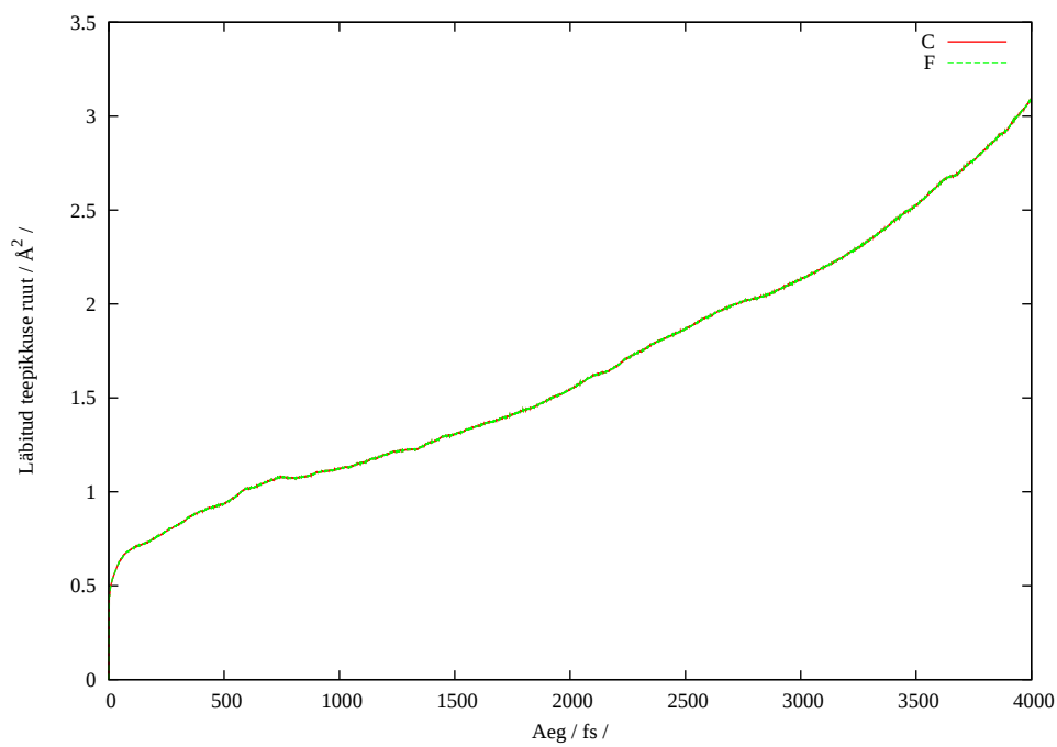
Joonis 5: Keskmise ruutnihke sõltuvus ajast
