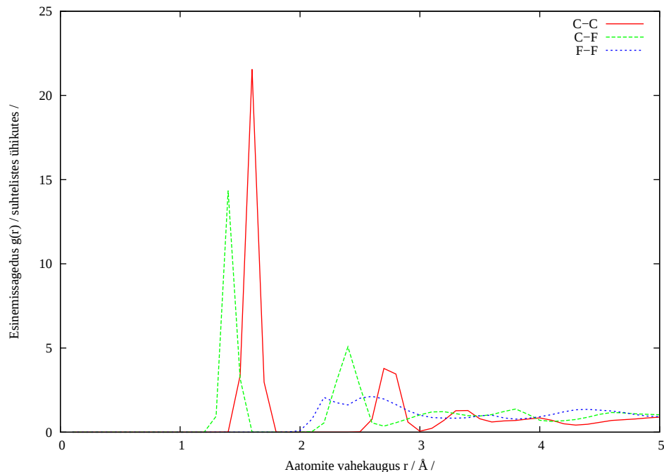
Joonis 4: Modelleeritud Tefloni radiaaljaotusfunktsioon
