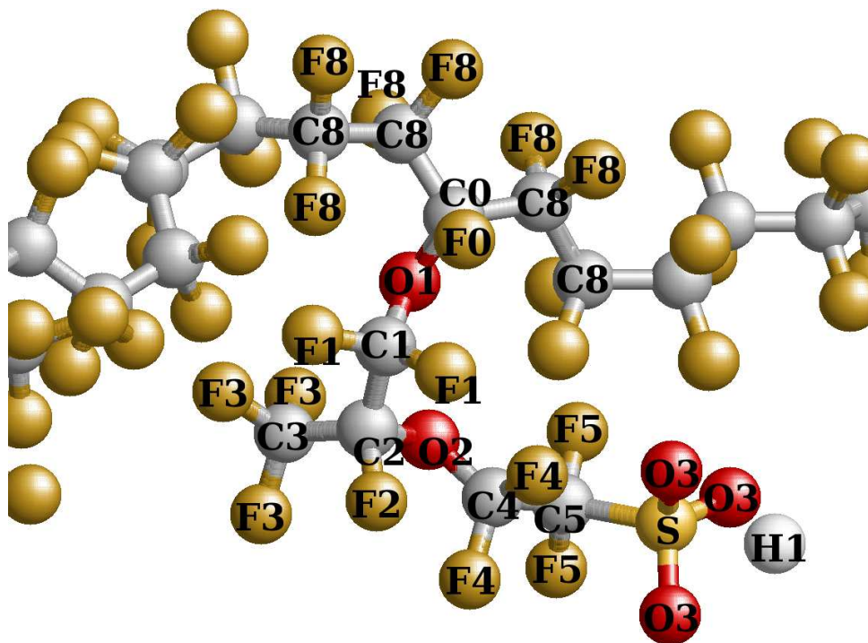
Joonis 1: Lõik nafioni® ahelast. Aatomid C8 ja F8 kuuluvad peaahelasse, ülejäänud kõrvalahelasse.
