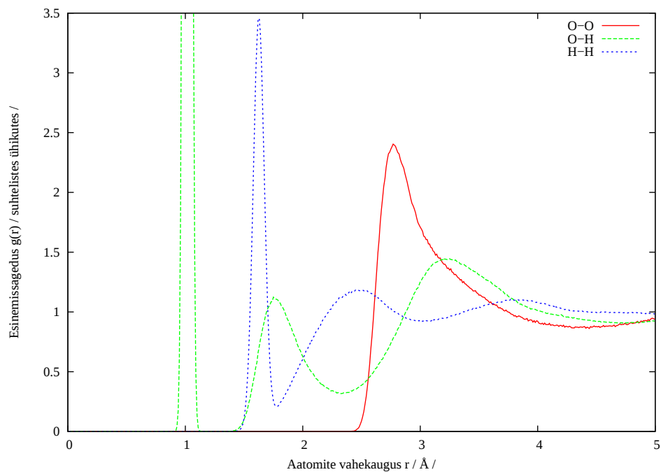
Joonis 5: Modelleeritud vee radiaaljaotusfunktsioonid
